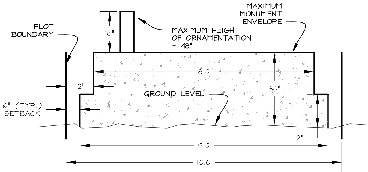
SECTION A-A
